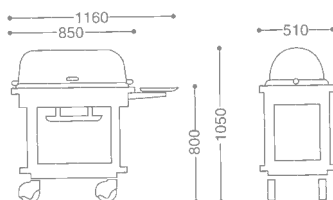
EUROPEAN ROAST BEEF SERVICE WAGON/OBLONG ヨーロッパ角ローストビーフワゴンA
