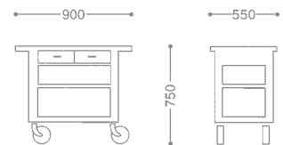
PRESTIGE SERVICE WAGON プレスステージサービスウゴン 0101 0090 ¥700,000 ● 18-8 ST.ST+WOOD ● FREE CASTER ● CHERRY WOOD+ URETHANE COATING
